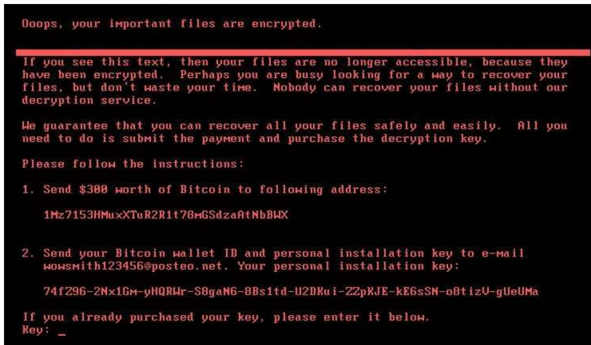
شکل ۱: سیستم آلوده
